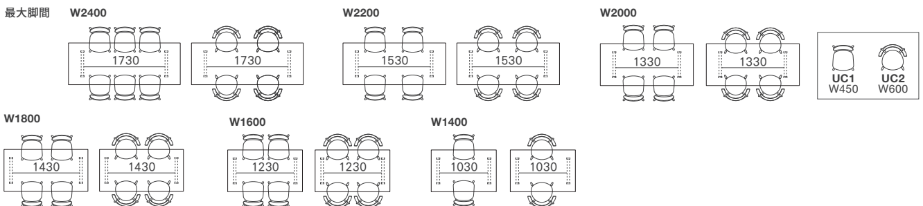
天板 穴位置 : 外側
